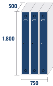
ECOV-25/3 PRO 39,1kg · 0,67m 3
