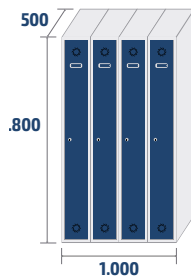
ECOV-25/4 PRO 50,3kg · 0,9m 3
