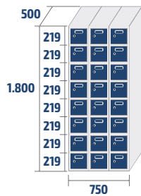
ECOZ-25/3 PRO 63,2kg · 0,67m 3
