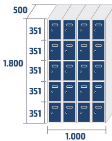
ECOP-25/4 PRO 71,8kg · 0,9m 3
