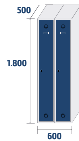
ECOV-30/2 PRO 30,2kg · 0,54m 3
