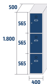
ECOM-40/1 PRO 24,2kg · 0,36m 3
