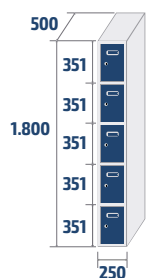
ECOP-25/1 PRO 21,7kg · 0,22m 3
