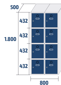
ECOC-40/2 PRO 45,4kg · 0,72m 3
