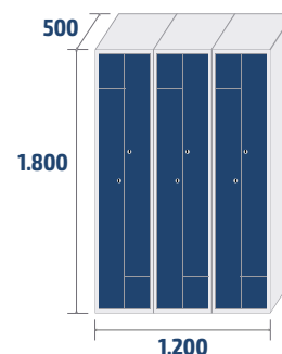
ECOL-40/3 PRO 72,3kg · 1,08m 3
