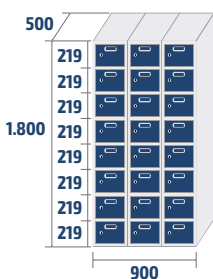
ECOZ-30/3 PRO 70,1kg · 0,81m 3
