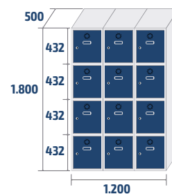
ECOC-40/3 PRO 65,1kg · 1,08m 3
