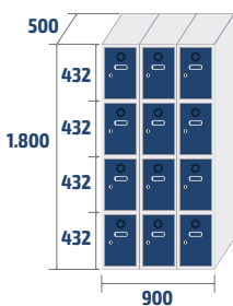
ECOC-30/3 PRO 54,9kg · 0,81m 3
