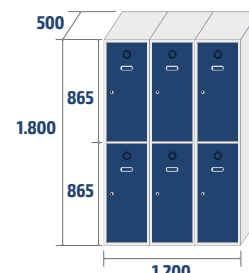
ECOT-40/3 PRO 59kg · 1,08m 3
