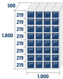
ECOZ-25/4 PRO 82,6kg · 0,9m 3
