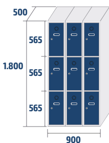
ECOM-30/3 PRO 51,6kg · 0,81m 3
