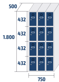
ECOC-25/3 PRO 50,4kg · 0,67m 3
