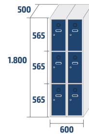
ECOM-30/2 PRO 36,4kg · 0,54m 3
