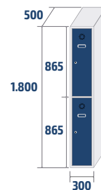
ECOT-30/1 PRO 19,1kg · 0,27m 3
