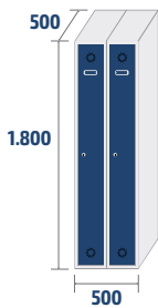
ECOV-25/2 PRO 27,9kg · 0,45m 3
