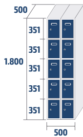
ECOP-25/2 PRO 38,4kg · 0,45m 3
