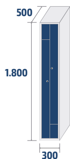
ECOL-30/1 PRO 24,4kg · 0,27m 3
