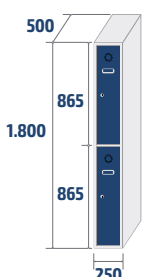
ECOT-25/1 PRO 18,4kg · 0,22m 3
