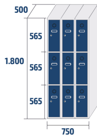
ECOM-25/3 PRO 47,7kg · 0,67m 3
