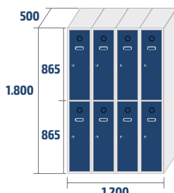
ECOT-30/4 PRO 61,4kg · 1,08m 3
