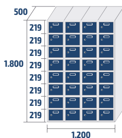
ECOZ-30/4 PRO 91,8kg · 1,08m 3
