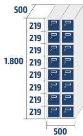
ECOZ-25/2 PRO 43,8kg · 0,45m 3
