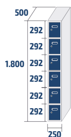
ECOB-25/1 PRO 22,6kg · 0,22m 3
