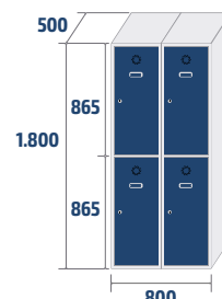
ECOT-40/2 PRO 41kg · 0,72m 3
