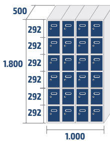
ECOB-25/4 PRO 75,4kg · 0,9m 3
