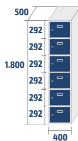
ECOB-40/1 PRO 28,1kg · 0,36m 3
