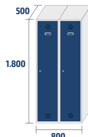
ECOV-40/2 PRO 35,1kg · 0,72m 3
